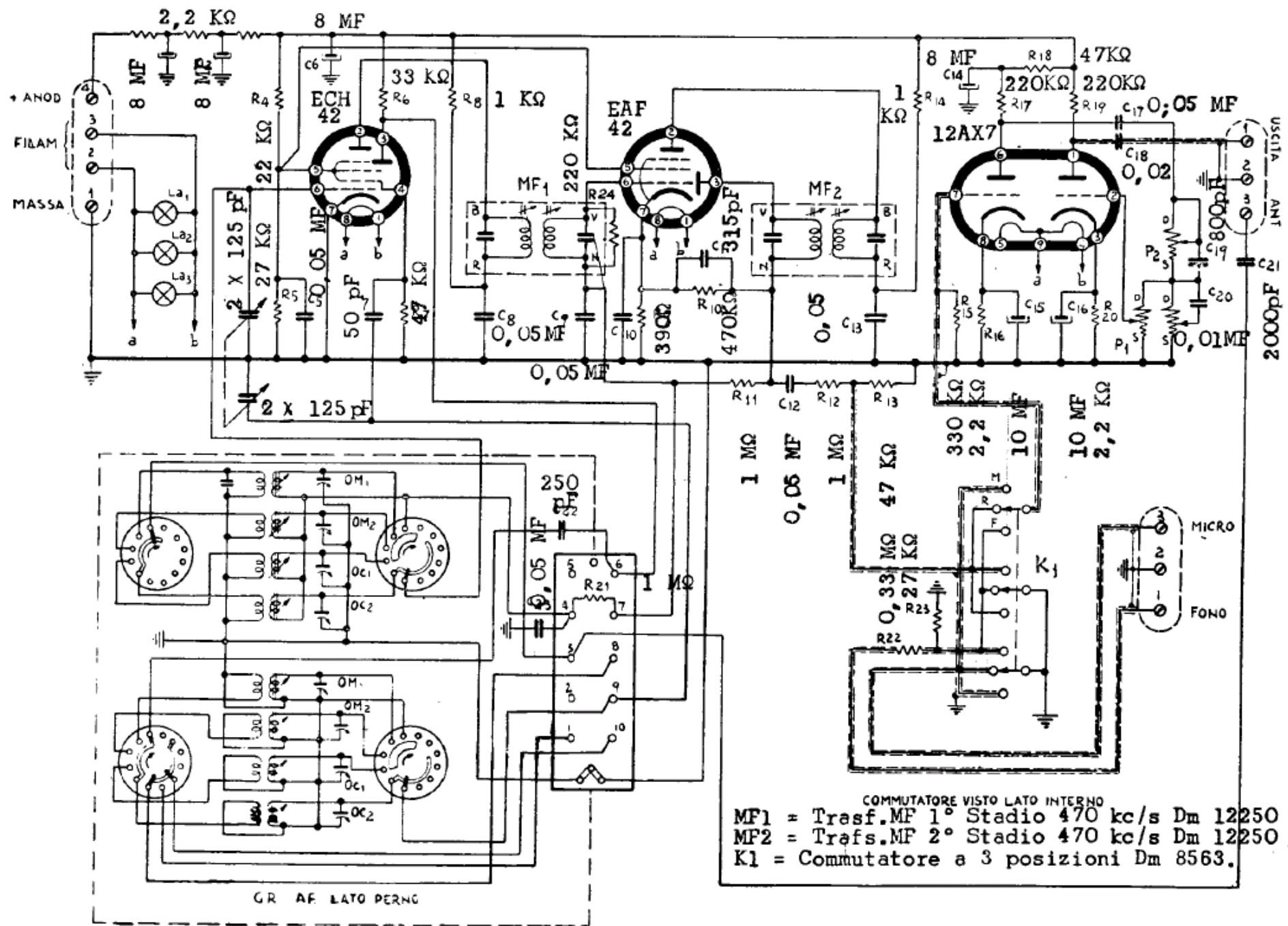
LESA - RADIOSINTONIZZATORE mod. RS/5. Due gamme onde medie: da 320 a 590 m e da 180 a 330 m. Due gamme OC: da 26 a 55 m e da 14 a 27 m.
